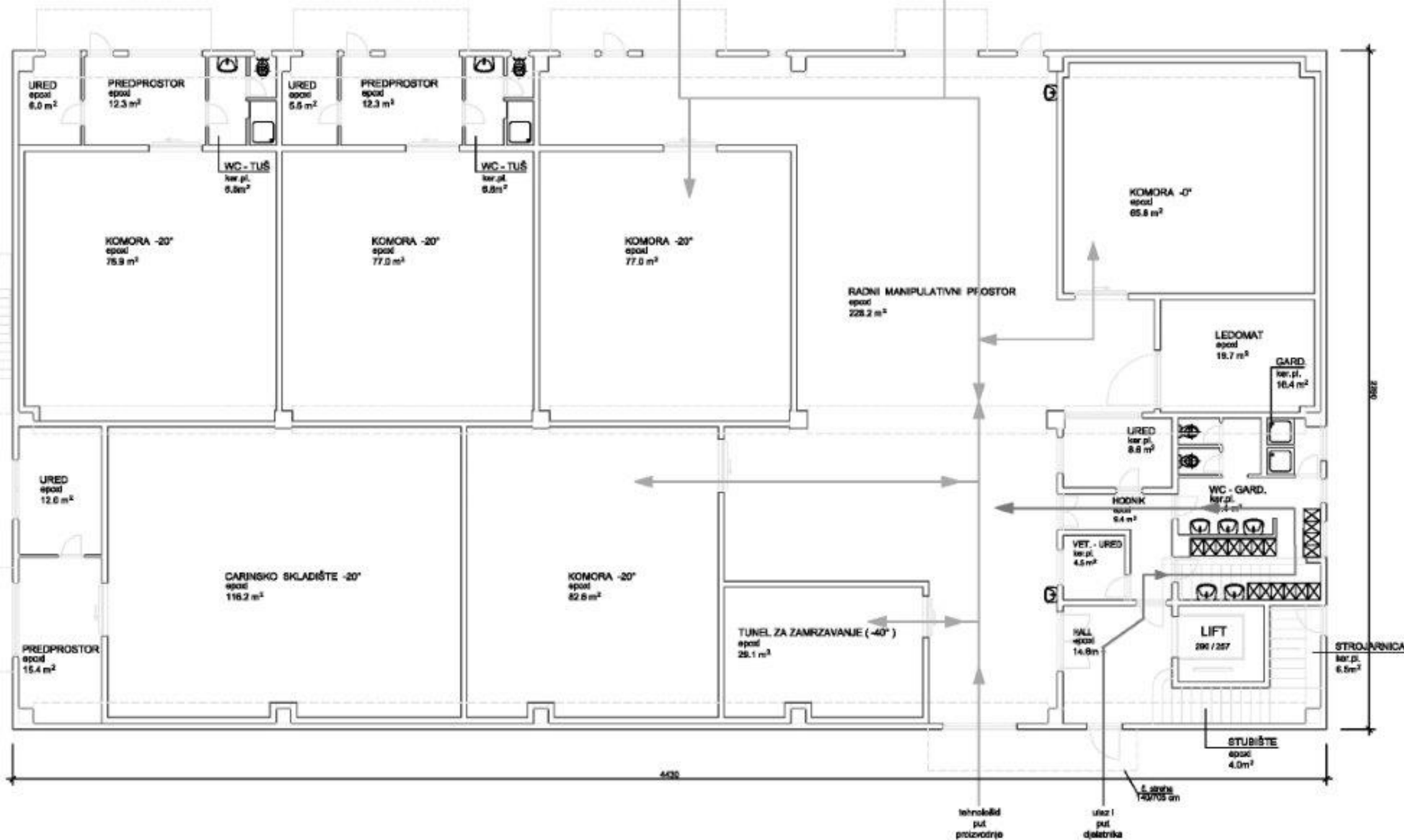
PRILOG 5 Tehnološki put proizvodnje u prizemlju
